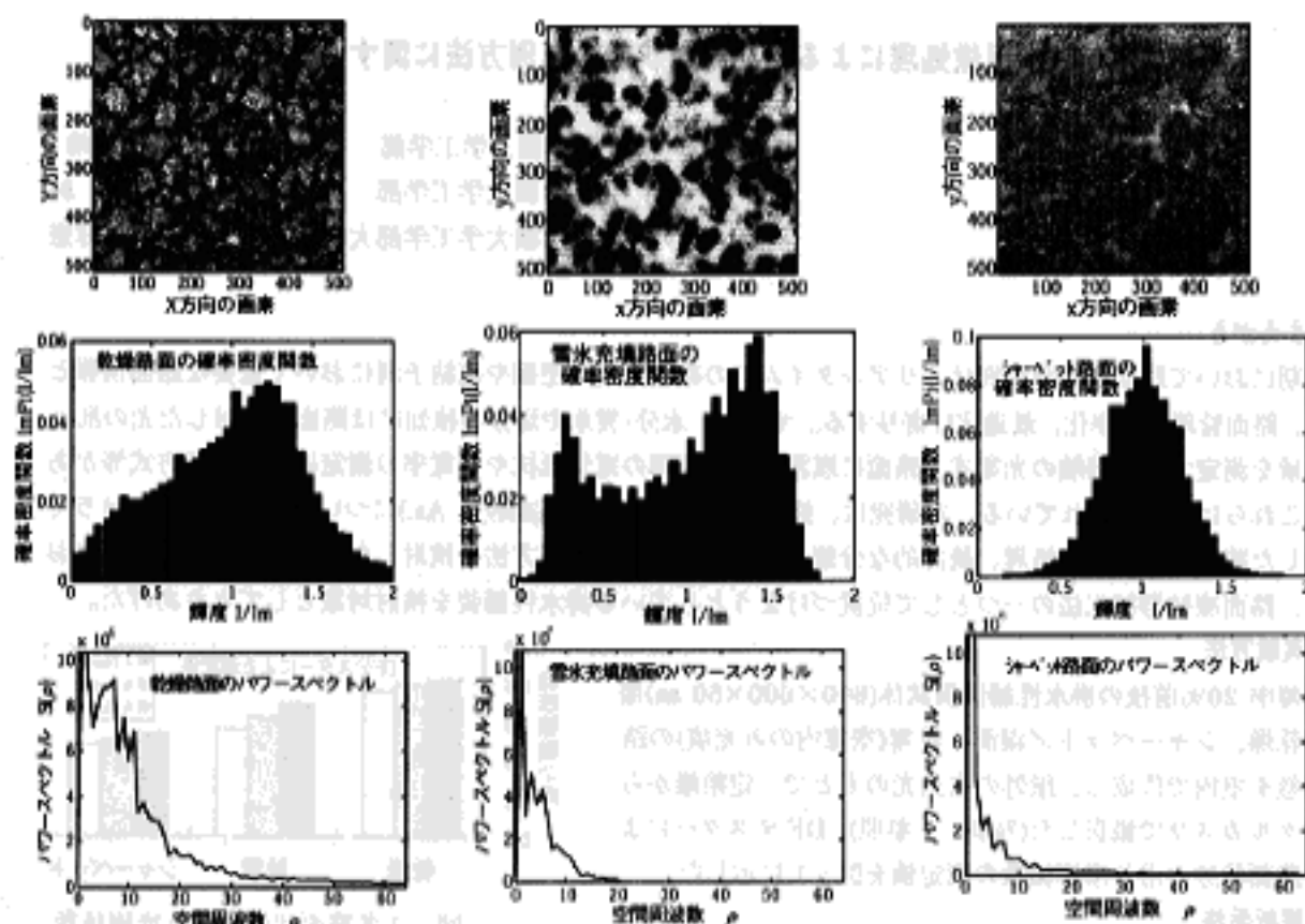
図-2 乾燥路面の写真(上)、密度関数(中)、パワースペクトル(下) 図-3 雪水充填路面の写真(上)、密度関数(中)、パワースペクトル(下) 図-4 シヤベット路面の写真(上)、密度関数(中)、パワースペクトル(下)
