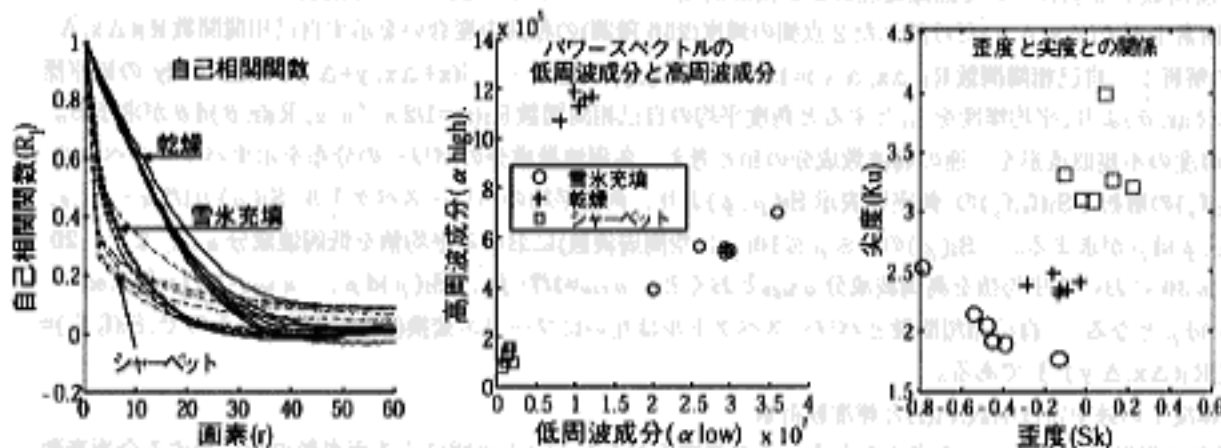
図-5 自己相関関数の分布 図-6 低・高周波数成分の分布 図-7 歪度と尖度の分布
