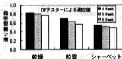
図-1 各路面状態の滑り摩擦係数
